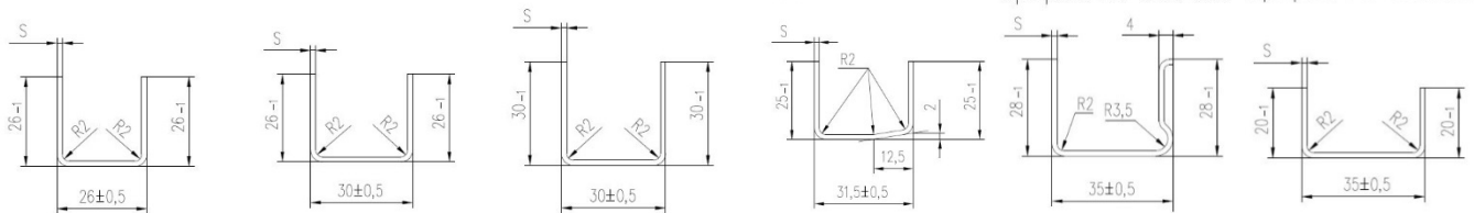
Профиль AV 26x26xS Профиль AV 30x26xS Профиль AV 30x30xS Профиль AV 31,5x25xS Профиль AV 35x28xS Профиль AV 35x20xS
